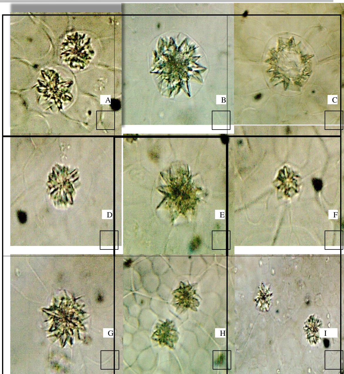
Figure 2. Druses observed in: A. Aglaonema sp., B. Alocasia macrorrhiza , C. Anthurium sp., D. Colocasia esculenta , E. Dieffenbachia seguine , F. Homalomena philippinensis , G. Philodendron sp., H. Spathiphyllumcommutatatum and I. Syngonium podophyllum . Magnification: 400x
